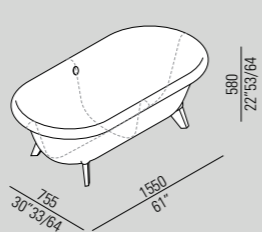
Ottocento small AVAS0967_
