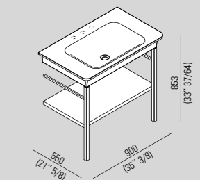
Novecento XL ACER 1071_
