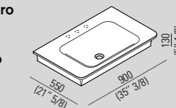
Novecento XL ACER 1070_
