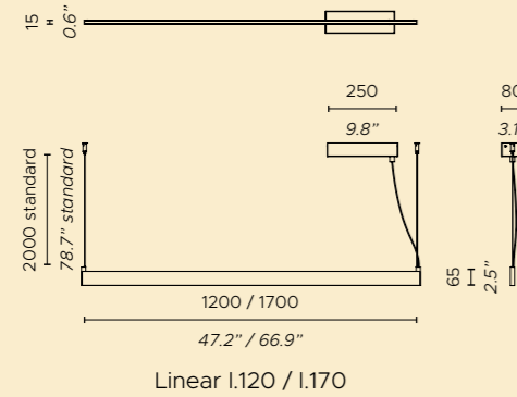
Linear I.120 / I.170
