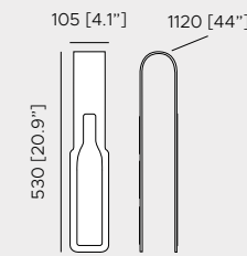
SEATS & SOFA FIXING / FISSAGGIO POLTRONE E DIVANI
