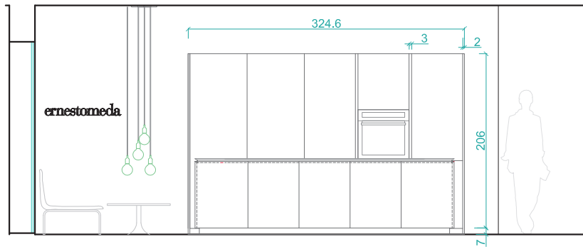
PROSPETTO FRONTALE
