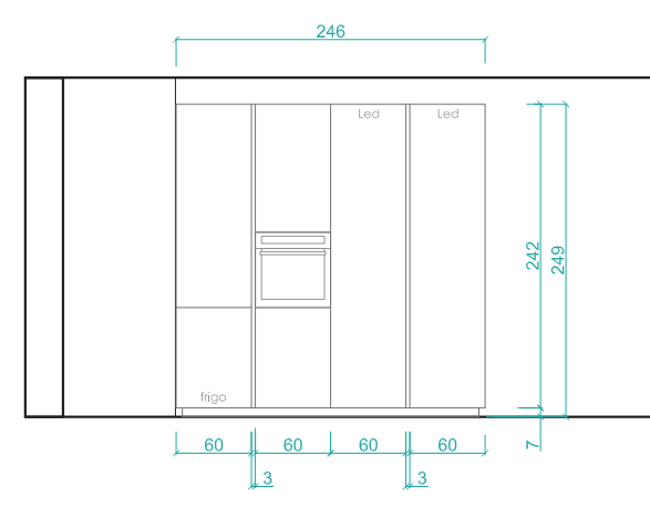
PROSPETTO COLONNE
