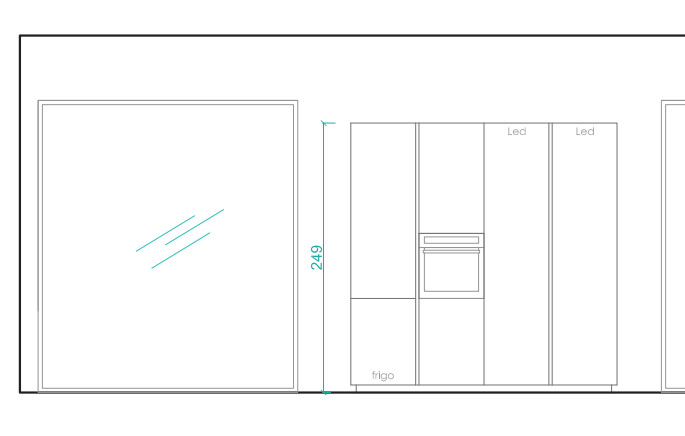
PROSPETTO COLONNE
