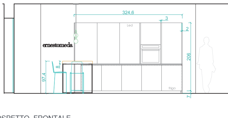
PROSPETTO FRONTALE
