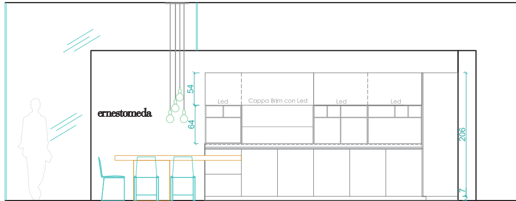
PROSPETTO BASI
