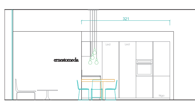
PROSPETTO COLONNE
