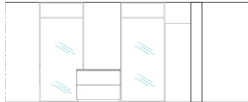
PROSPETTO LATERALE
