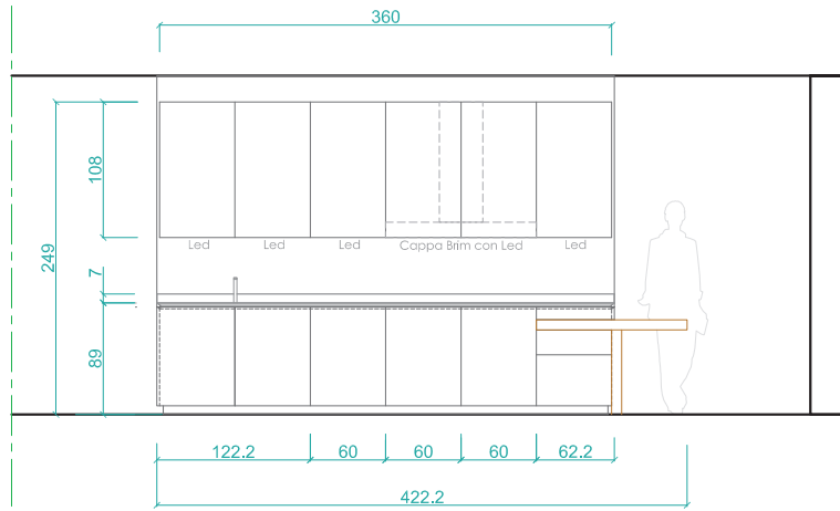
PROSPETTO BASI
