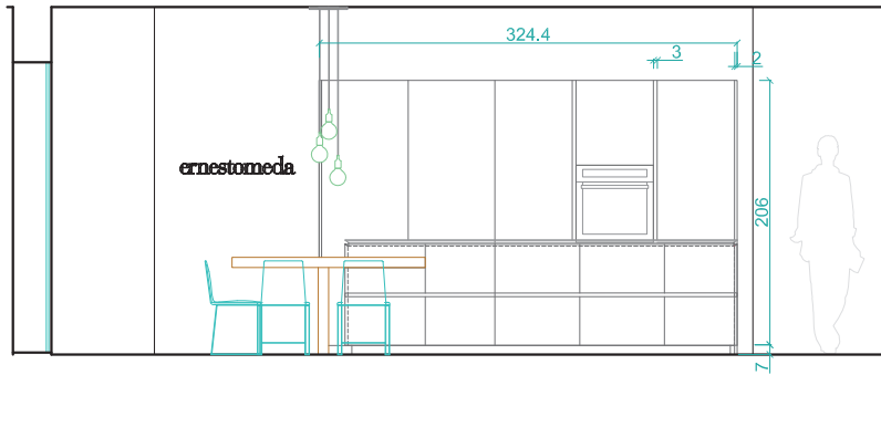
PROSPETTO FRONTALE
