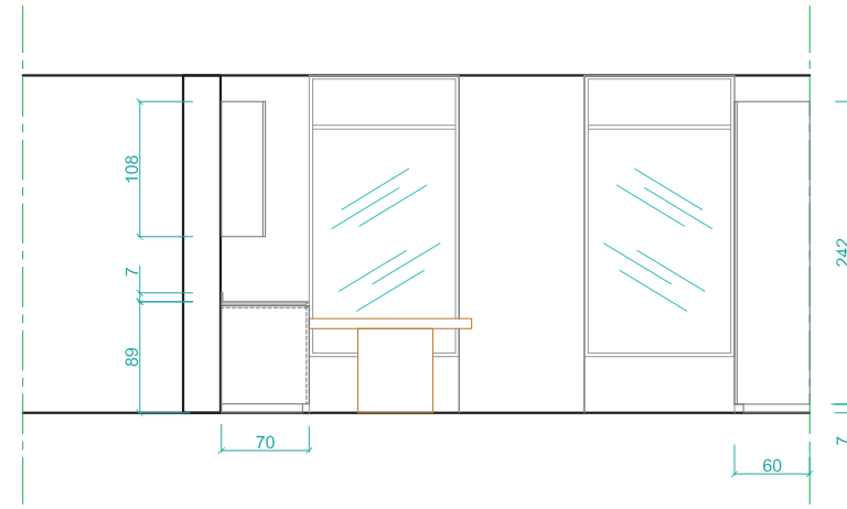
PROSPETTO LATERALE
