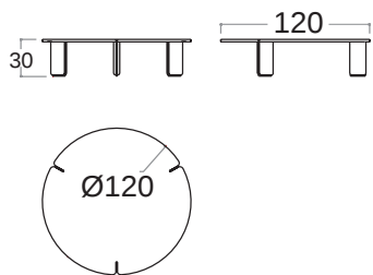
CENTRAL ROUND TABLE Ø 120 TAVOLINO ROTONDO Ø 120
