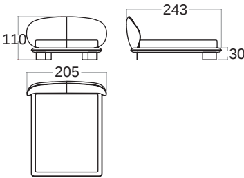
BED X SPRING 160X200 LETTO PER RETE 160X200
