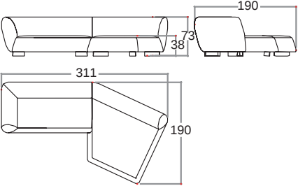
SOFA COMPOSITION 2 COMPOSIZIONE DEL DIVANO 2
