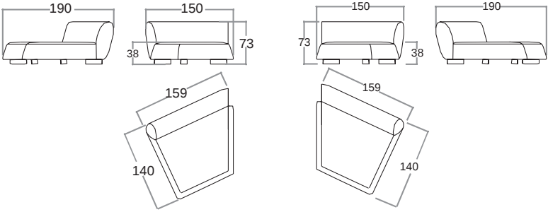
SIDE ELEMENT RH - LH WITHOUT ARMREST FINALE INCLINATO DX-SX SENZA BRACCIOLO
