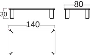
RECTANGULAR COFFEE TABLE 140x80 GEA TAVOLINO RETTANGOLARE 140x80
