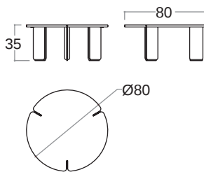
COFFEE TABLE Ø 80 TAVOLINO ROTONDO Ø 80
