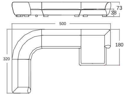
SOFA COMPOSITION 1 COMPOSIZIONE DEL DIVANO 1
