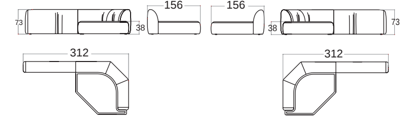
CORNER ELEMENT RH - LH ANGOLARE DX SX
