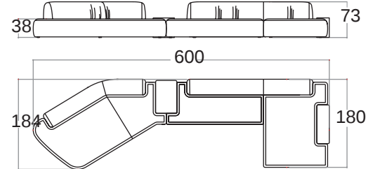
SOFA COMPOSITION 1 DUNE COMPOSIZIONE DEL DIVANO 1 DUNE
