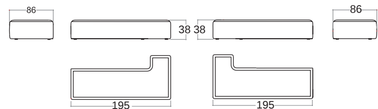
END ELEMENT RH - LH FINALE DX SX
