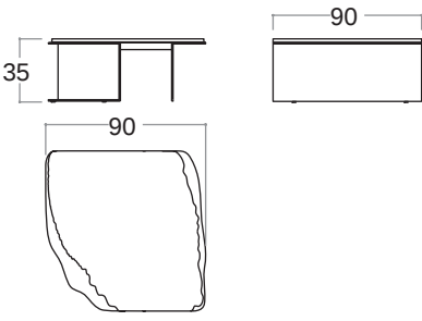
SQUARE COFFEE TABLE 90 TAVOLINO QUADRATO 90
