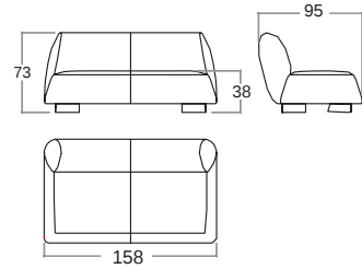
SOFA 2 SEATER WITHOUT ARMREST DIVANO 2 POSTI SENZA BRACCIOLI
