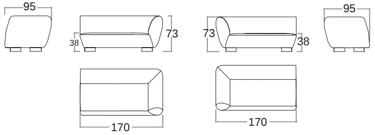
END ELEMENT WITH RH - LH ARMREST FINALE INCLINATO DX-SX CON BRACCIOLO
